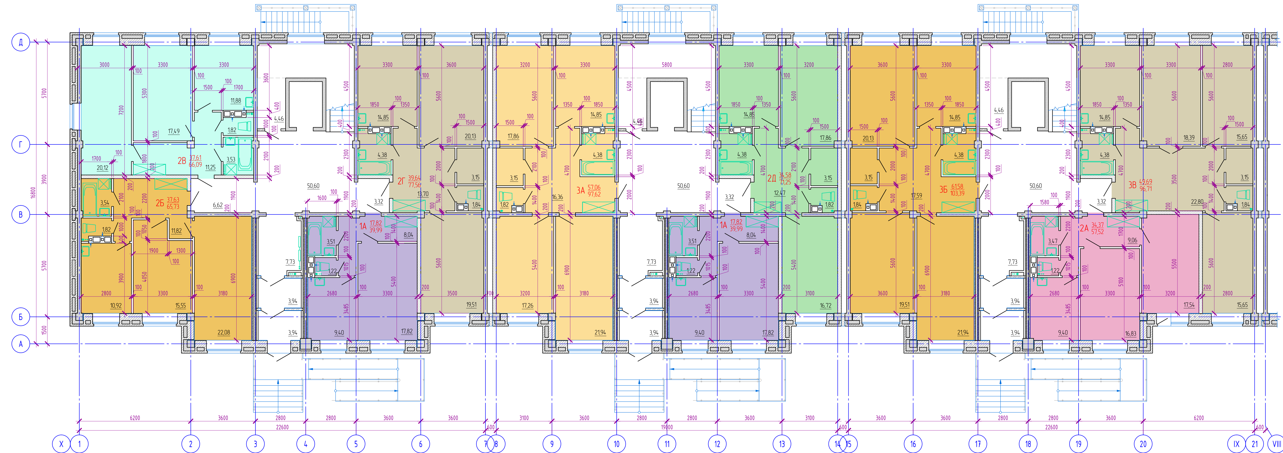
Объемно-планировочные показатели на блок-секцию
